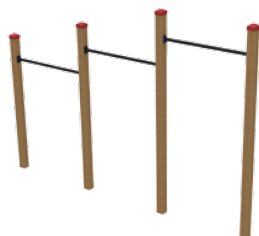
163 BARRE DI TRAZIONE L. 315cm - P. 9cm - H 220cm
