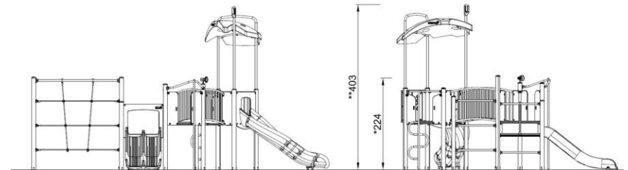
PCE206002 1:100
