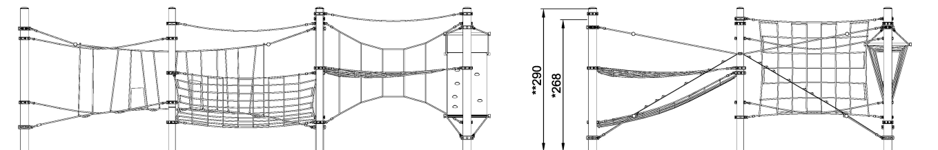
COR101301 1:100
