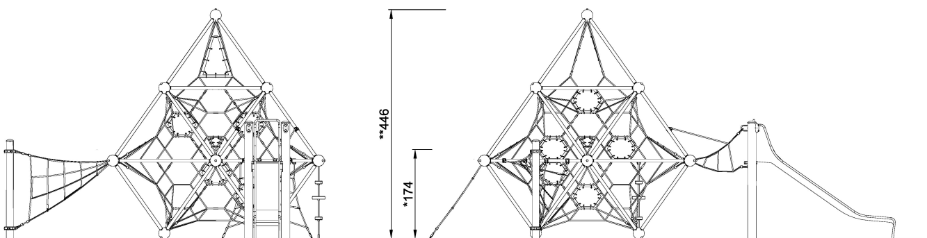
COR105131 1:100
