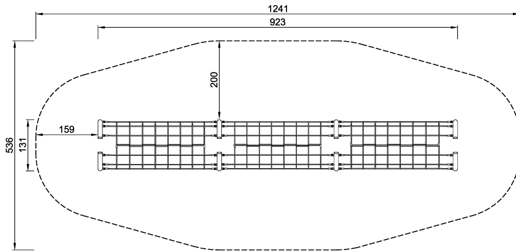
COR650901-xx01 *275cm **275cm **54.8m 2 1:100
