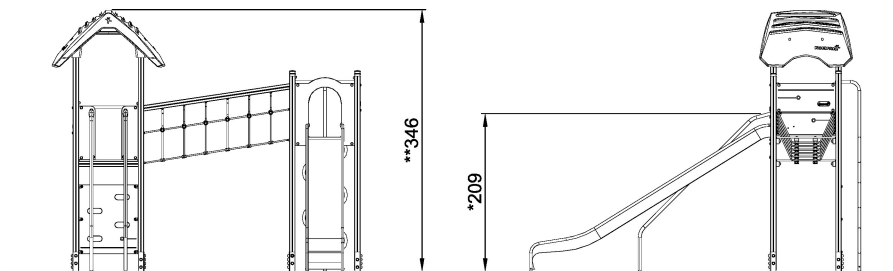
KPL201502 1:100
